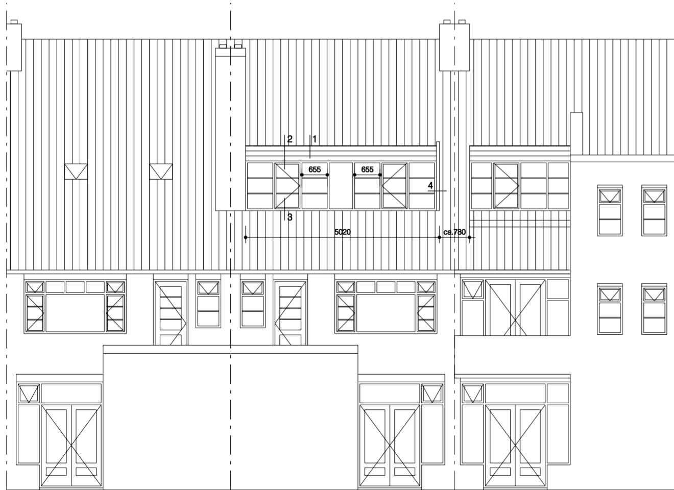
achtergevel gewijzigd
