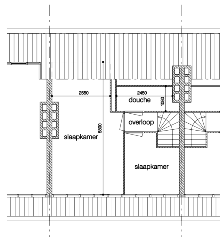
zolder bestaand
