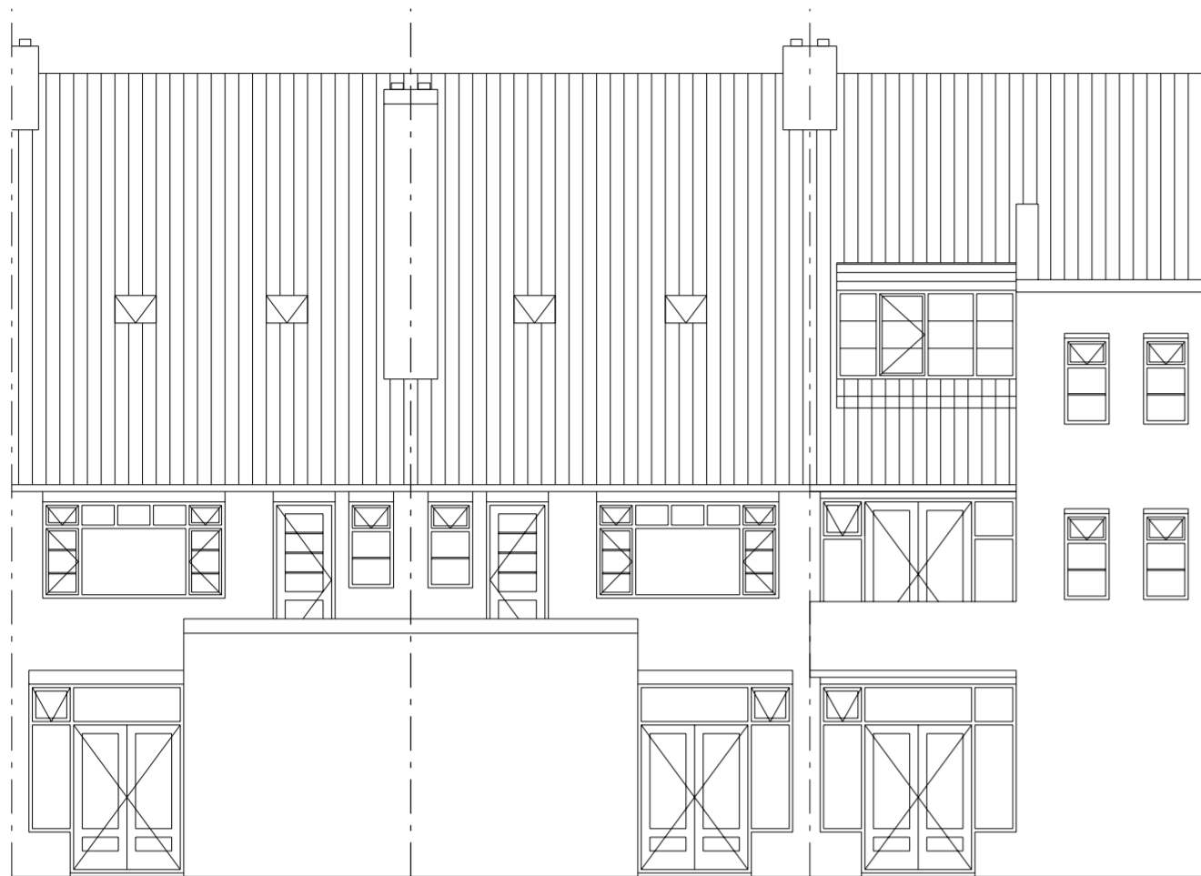
achtergevel bestaand
