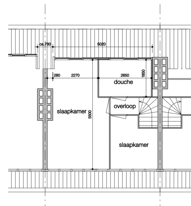
zolder gewijzigd
